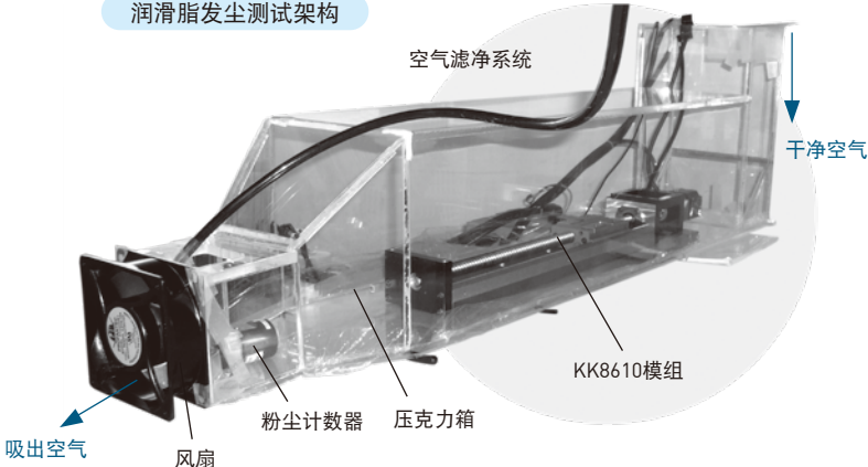
润滑脂发尘测试架构
