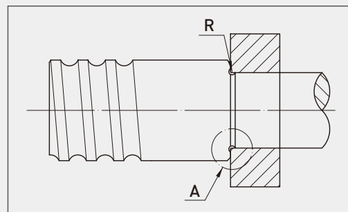
图4.10 轴承承靠面的逃槽
