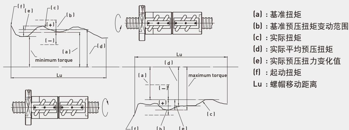
图 4.21 预压扭矩量测图
