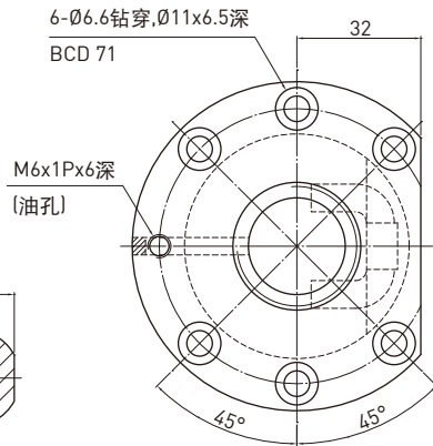
D-D 视图
