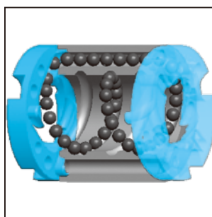
图3.6 端盖回流方式
