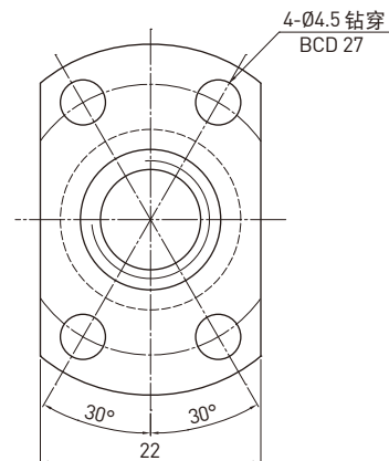
D-D 视图
