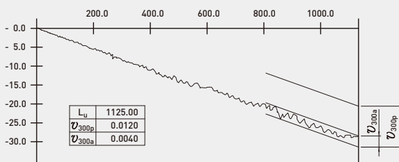
任意300mm长度内的导程变化
