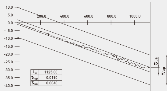
有效行程 L_u 内的导程变动
