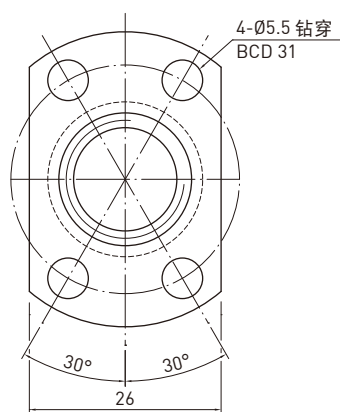
D-D 视图
