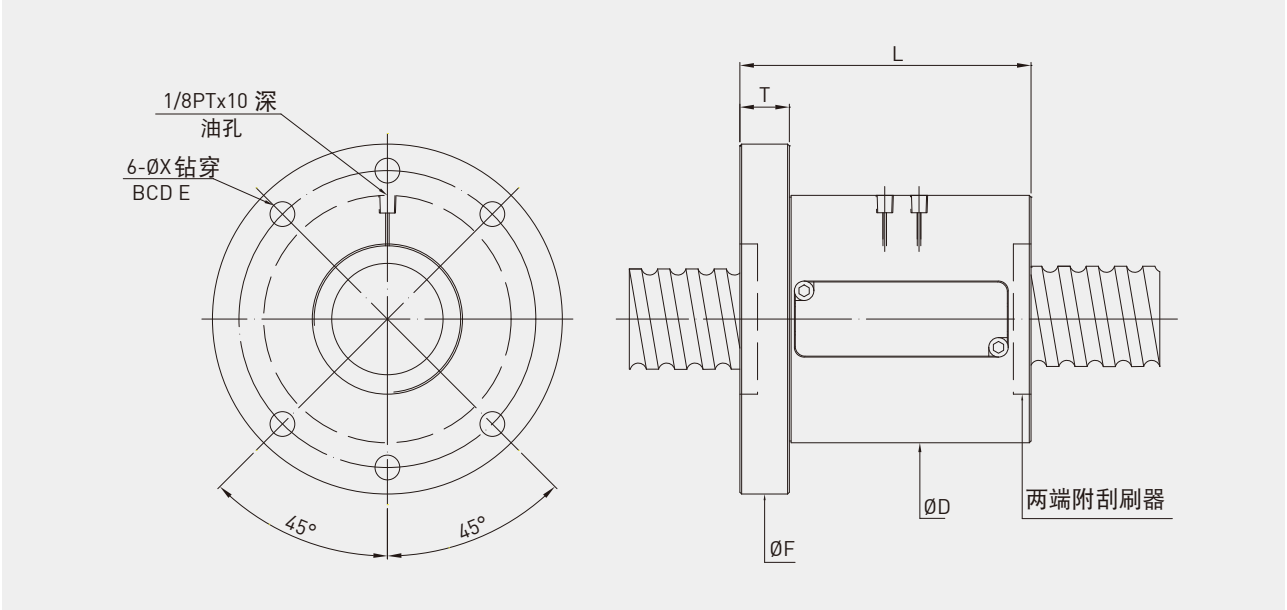
外塞式重负荷滚珠丝杠规格表 (FSS型)
