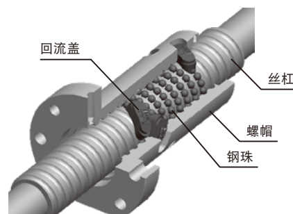
图3.2 内循环滚珠丝杠
