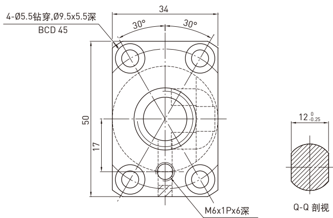
D-D 视图
