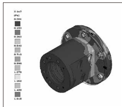
图8.10 Cool Type滚珠丝杠的有限元素分析
