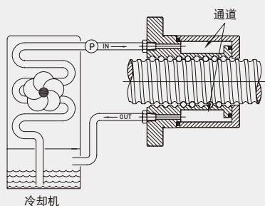
图 8.8 Cool type II 与冷却机示意图
