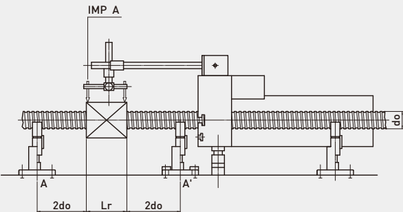
T7: 量测方形螺帽平面相对于AA’ 的平行度 (此量测距离是根据DIN 69051及JIS B1192)
