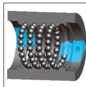
图3.7 Super S 回流方式
