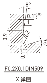
X 详图
