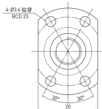
D-D 视图
