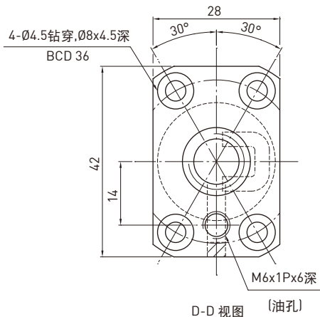
D-D 视图 (油孔)
