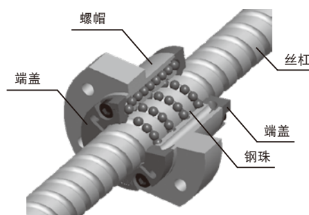
图3.3 端盖式滚珠丝杠
