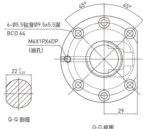
D-D 视图
