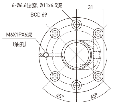
D-D 视图
