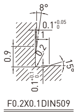
X 详图
