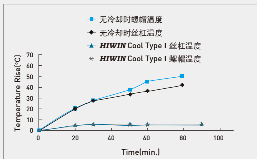
图8.4 高速运转下 Cool type I 滚珠丝杠的温升表现
