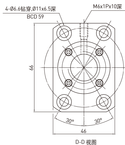
Q-Q 剖视
