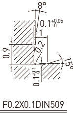
X 详图
