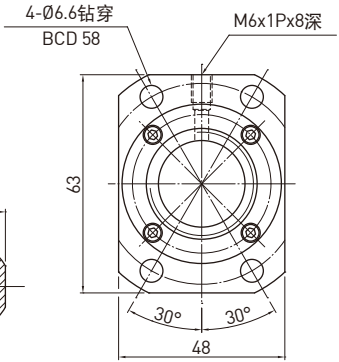
D-D 视图
