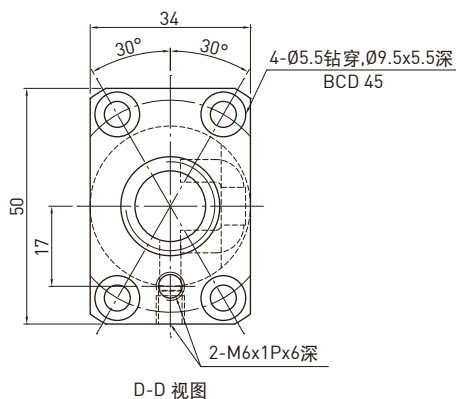
D-D 视图
