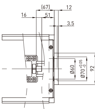
电机连接法兰F2
