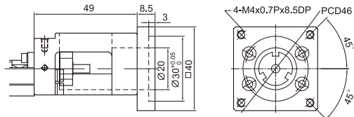
电机连接法兰 F2
