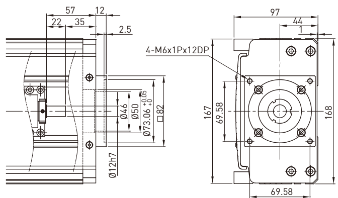
电机连接法兰 F4
