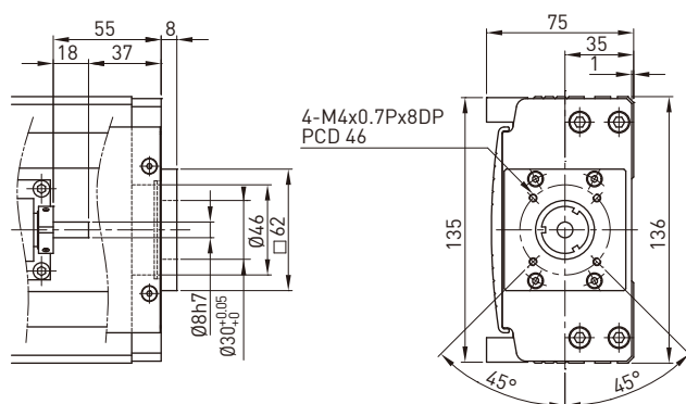
电机连接法兰F2
