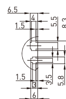
E 详图
