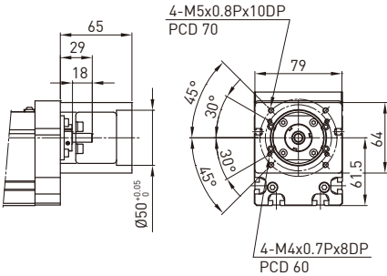
电机法兰 F0
