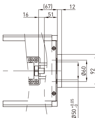
电机连接法兰F1
