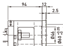
电机连接法兰 F4
