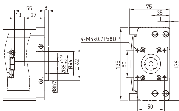
电机连接法兰F5
